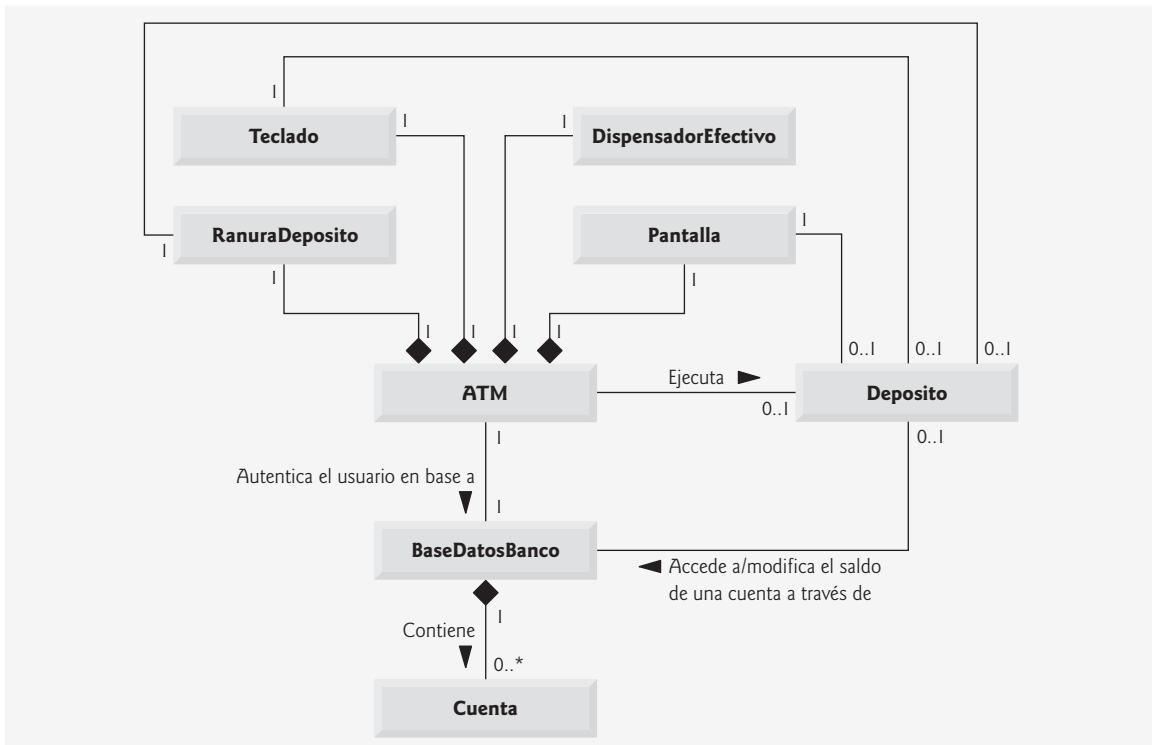
Figura 3.26 | Diagrama de clases para el modelo del sistema ATM, incluyendo la clase Depósito.
