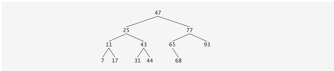
Figura 17.16 | Árbol de búsqueda binario que contiene 12 valores.
