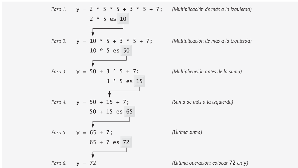
Figura 2.13 | Orden en el cual se evalúa un polinomio de segundo grado.
