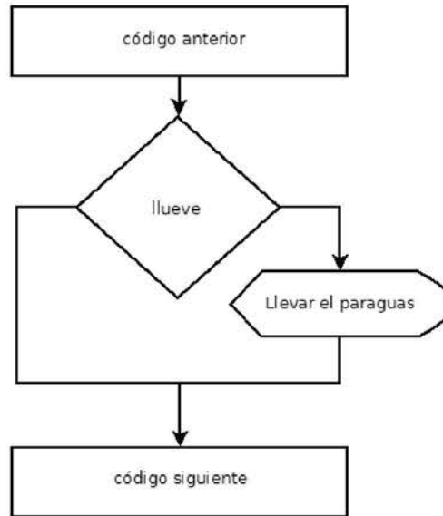
Figura 6-1. Diagrama de un condicional simple.
