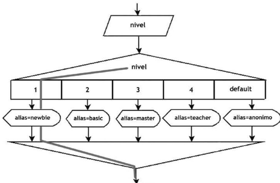
Figura 6-6. Diagrama de un switch con sus caminos excluyentes.
