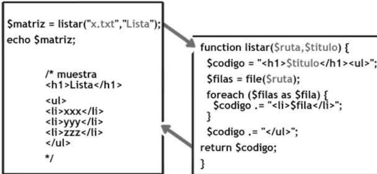
Figura 9-4. Función con más de un parámetro de entrada.
