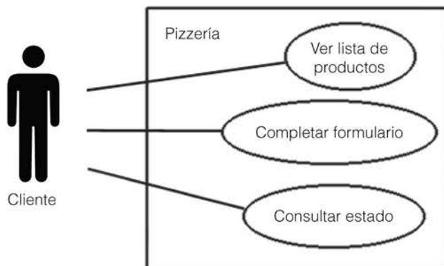
Figura 13-13. Diagrama de casos de uso del Cliente.
