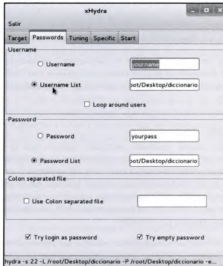
Imagen 03.11: Credenciales en Hydra.
