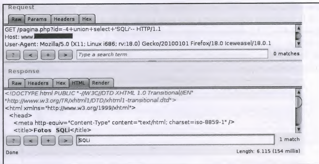
Imagen 05.14: Imprimiendo SQLi en el HTML.
