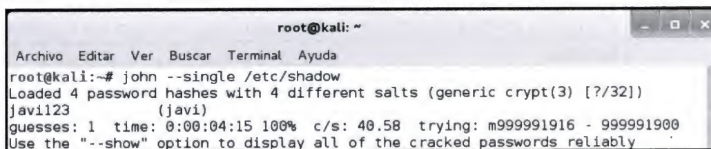
Imagen 03.14: Johntheripper modo single crack.
