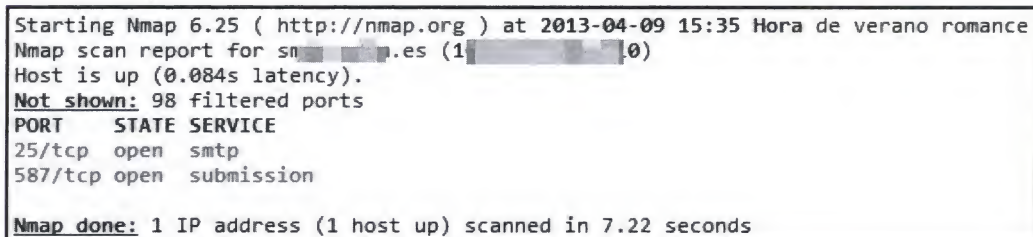
Imagen 02.24: Descubrimiento del servicio SMTP con nmap .
