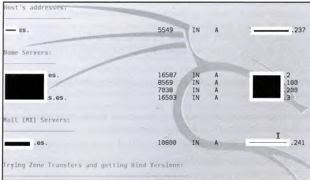
Imagen 02.23: Detección del servidor de correo con dnsenum .
