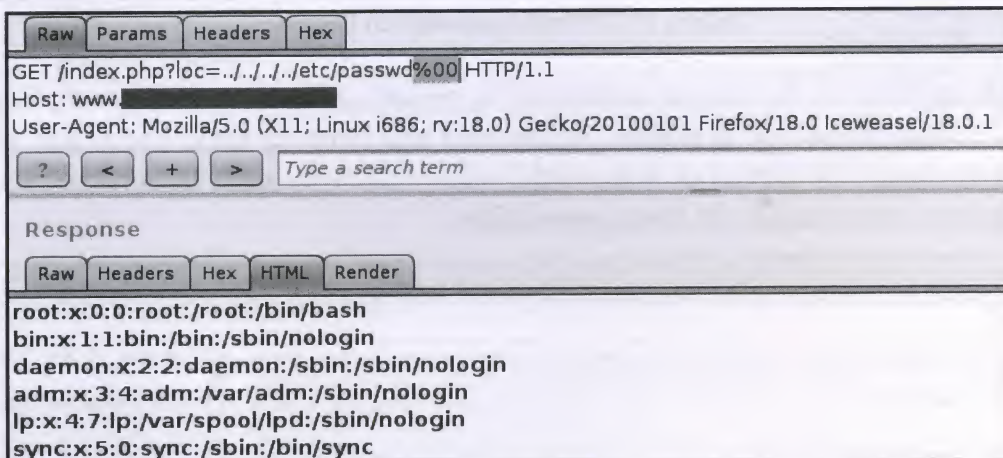
Imagen 05.22: Agregando el byte nulo para romper extensiones.
