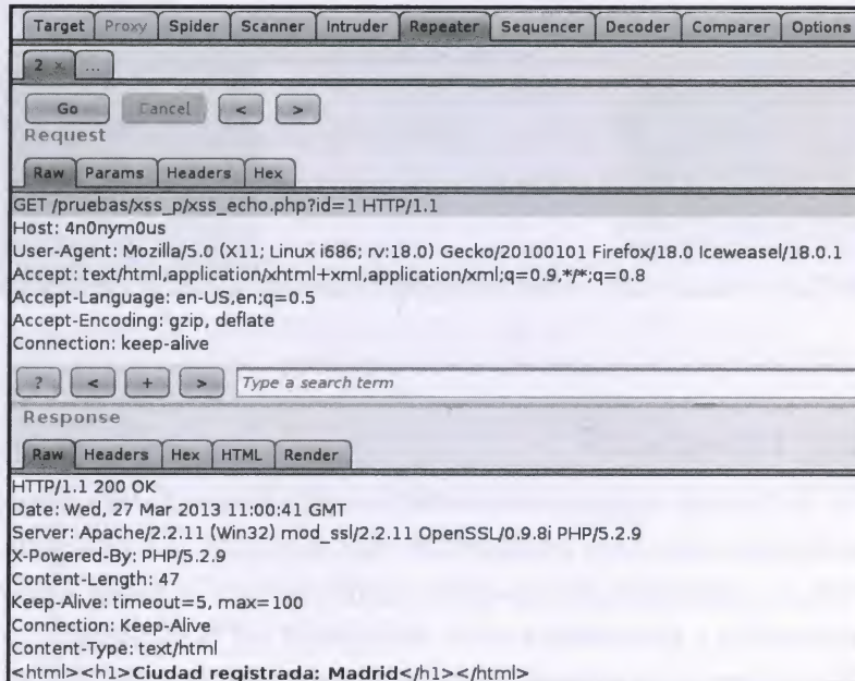
Imagen 05.07: Extracción de la ciudad de la base de datos.
