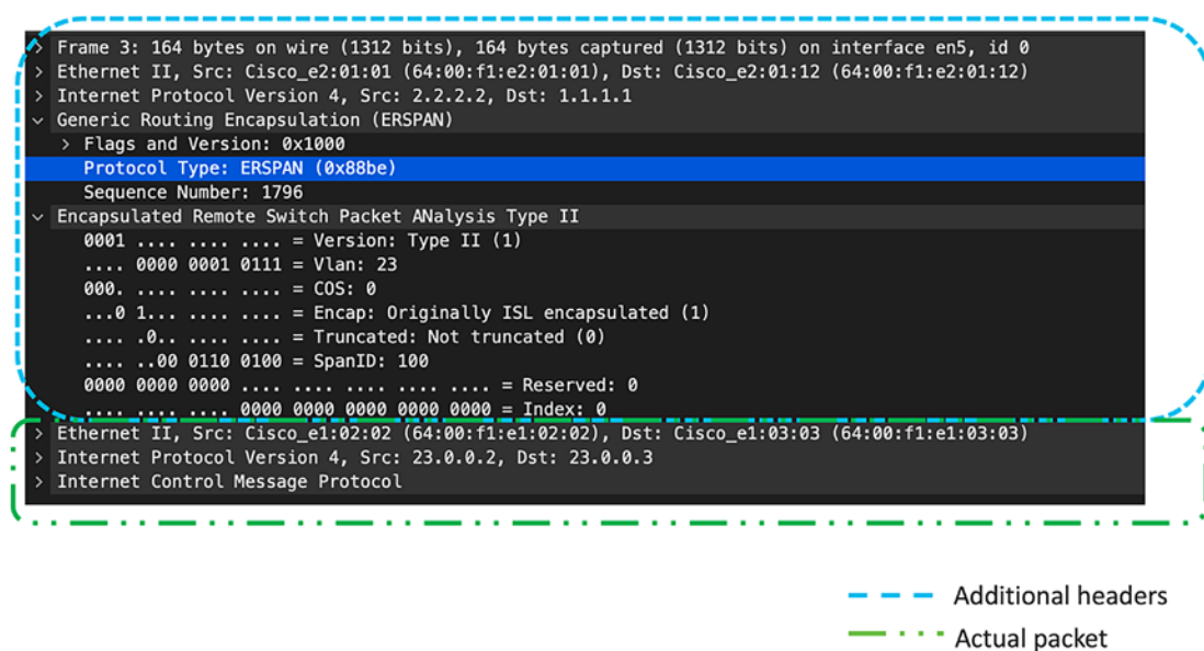
Figure 2-3. ERSPAN header
